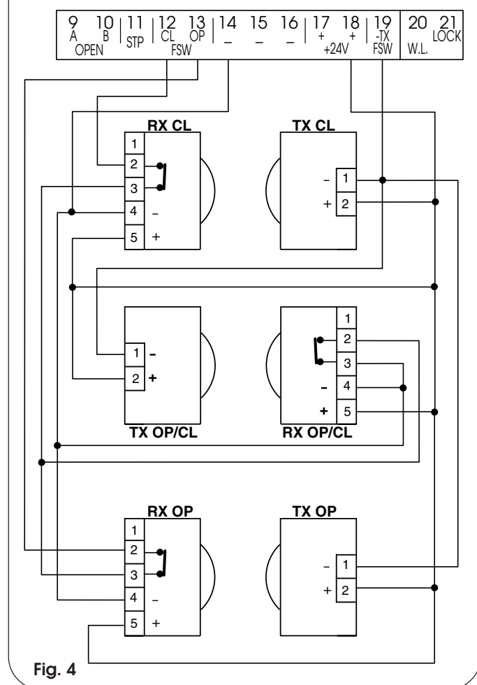
Connexion d'une paire de photocellules en fermeture, d'une paire de photocellules en ouverture et d'une paire de photocellules en ouverture/fermeture (schéma préconisé)
